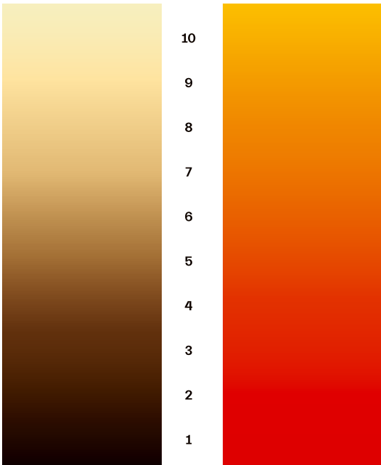
Eumelanin
